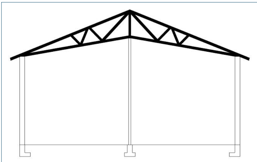
Konstruksjonsprinsipp for elementlaft.
