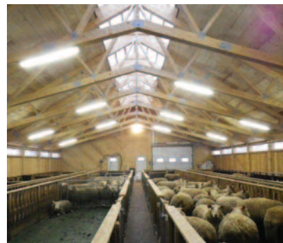
Sauefjøs med bæresystem av prefabrikkerte takstoler.
