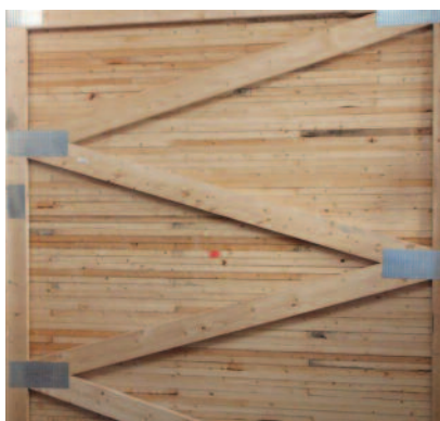
Vindavstiving, fagverk med spikerplater montert i tak.
