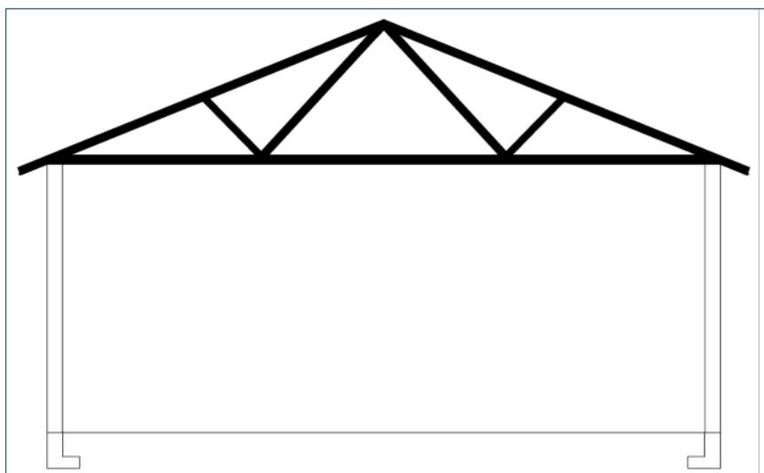
Konstruksjonsprinsipp for bindingsverk med takstoler.
