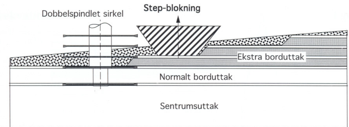
Fig. 7. To-spindlet flerblad sirkel med stepblokning.
