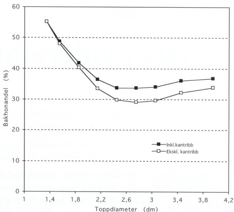
Figur 2. Potensial i bakhon for uttak av ekstra sidebord.
