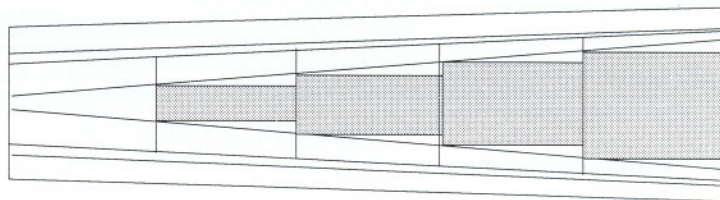
Figur 6. Kapping for kanting ved kasseborduttak gir øket utbytte.
