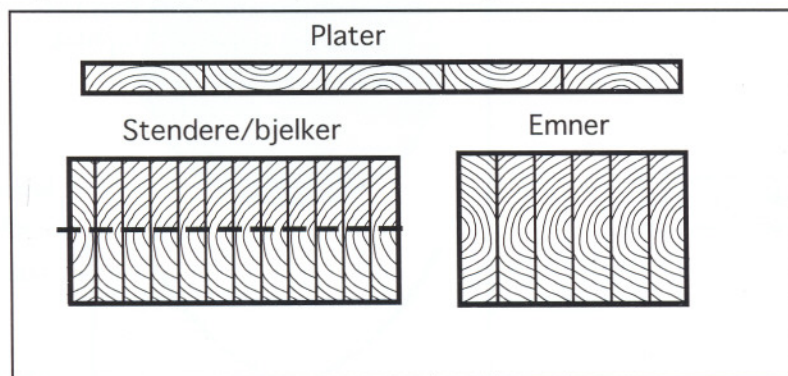
Fig. 8. Eksempel på limtreprodukter basert på sidebord.
