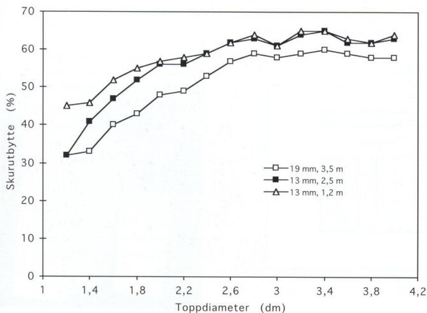
Figur 5. Skurutbytte avhengig av toppdiameter ved 3 forskjellige typer borduttak.
