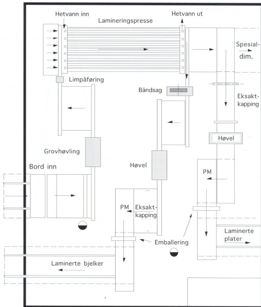
Figur 9. Eksempel på produksjonsopplegg for fremstilling av laminerte stendere, bjelker, emner og plater basert på 2,5 m bord.
