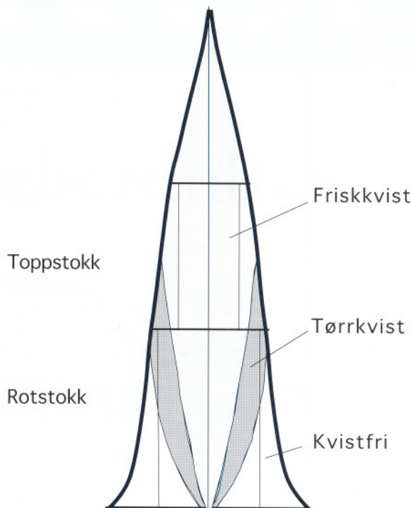
Figur 4. Kvistfordelingen i en furustamme (etter Kärkinen).
