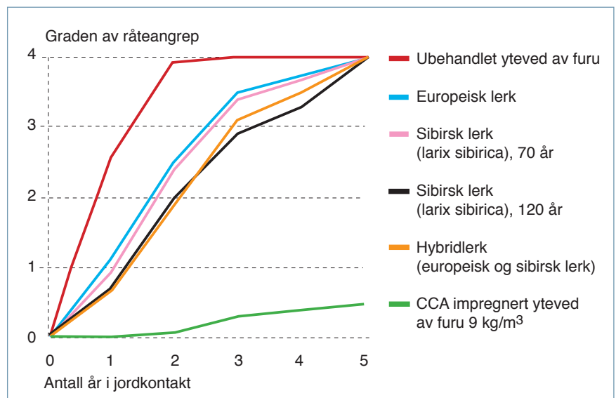
Figur 4. Råteutvikling i bakken for noen lerkarter, samt uimpregnert og impregnert yteved av furu gjennom 5 år. (Rapp, A.O, Viitanen, H & Nilsson, T 2002).
